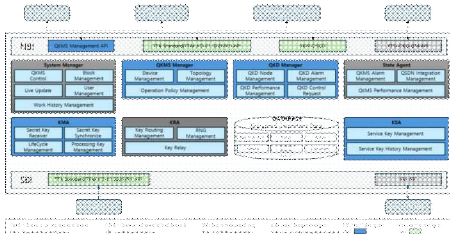
<QKMS 기반 QKD망 운용 SW 구성도>
