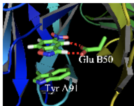
단백질-리간드 상호작용
